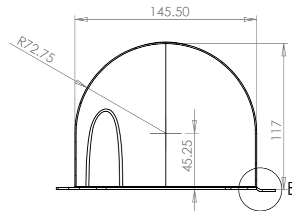
SECTION A-A SCALE 1 : 3
